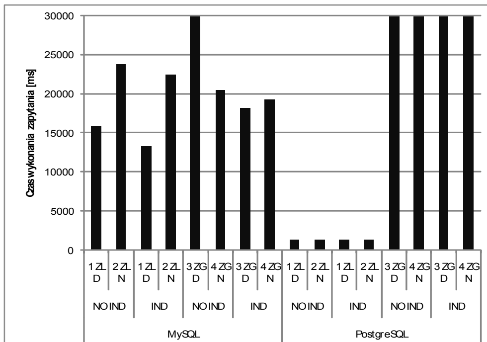
Rys. 5. Wyniki testów w ujęciu celu normalizacji dla niższych wartości Fig. 5. View of the impact of normalization for the lower values
