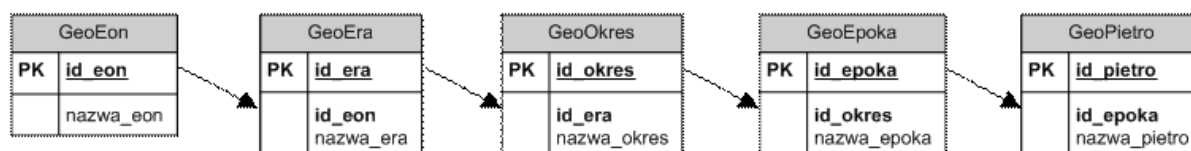
Rys. 1. Znormalizowany schemat tabeli geochronologicznej Fig. 1. Standardized schema of the geochronologic table
