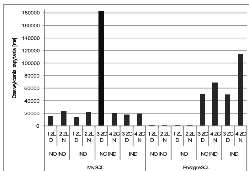
Rys. 4. Wyniki testów w ujęciu celu normalizacji Fig. 4. View of the impact of normalization
